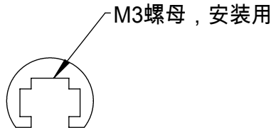
局部视图 A 比例 2 : 1
