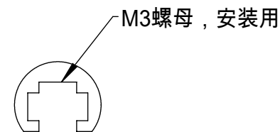
局部视图 A 比例 2 : 1
