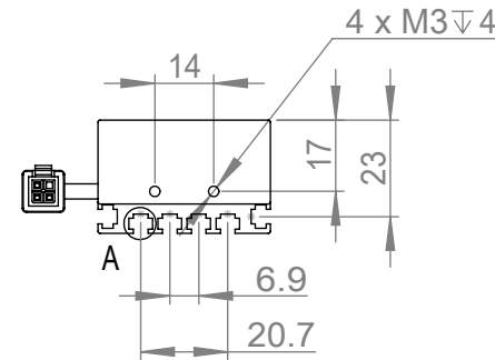
局部视图 A 比例 2 : 1
